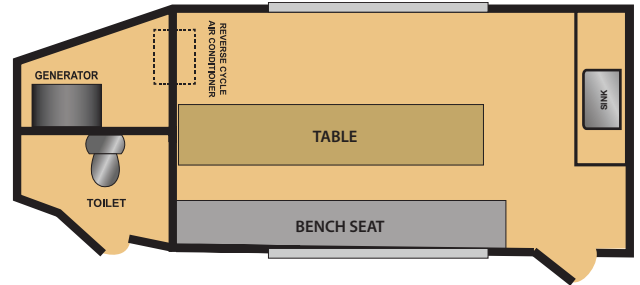
MTE Floorplan
